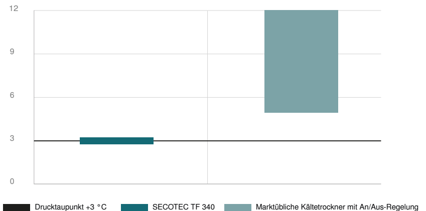
Trocknungsgrad als mittlerer Drucktaupunkt in °C
