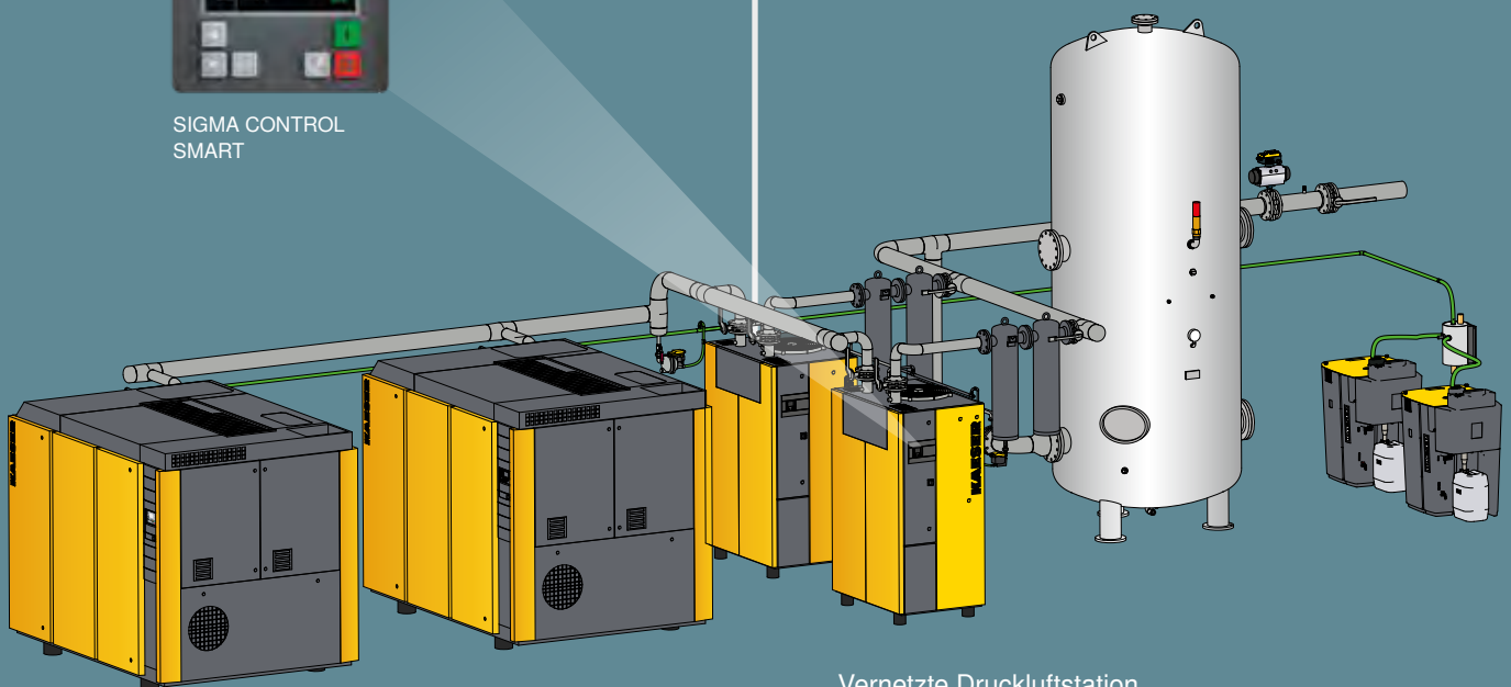
Vernetzte Druckluftstation
